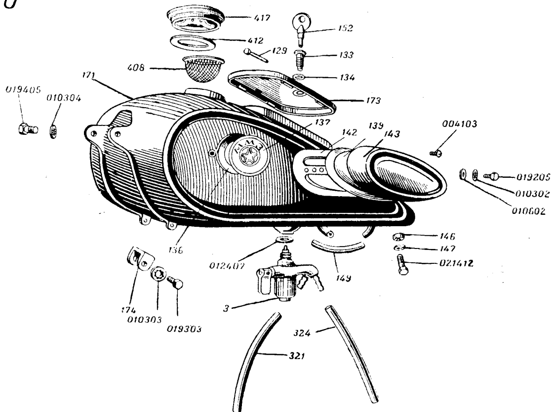
Рис. 8 ГРУППА 7210. БЕНЗИНОВЫЙ БАК
