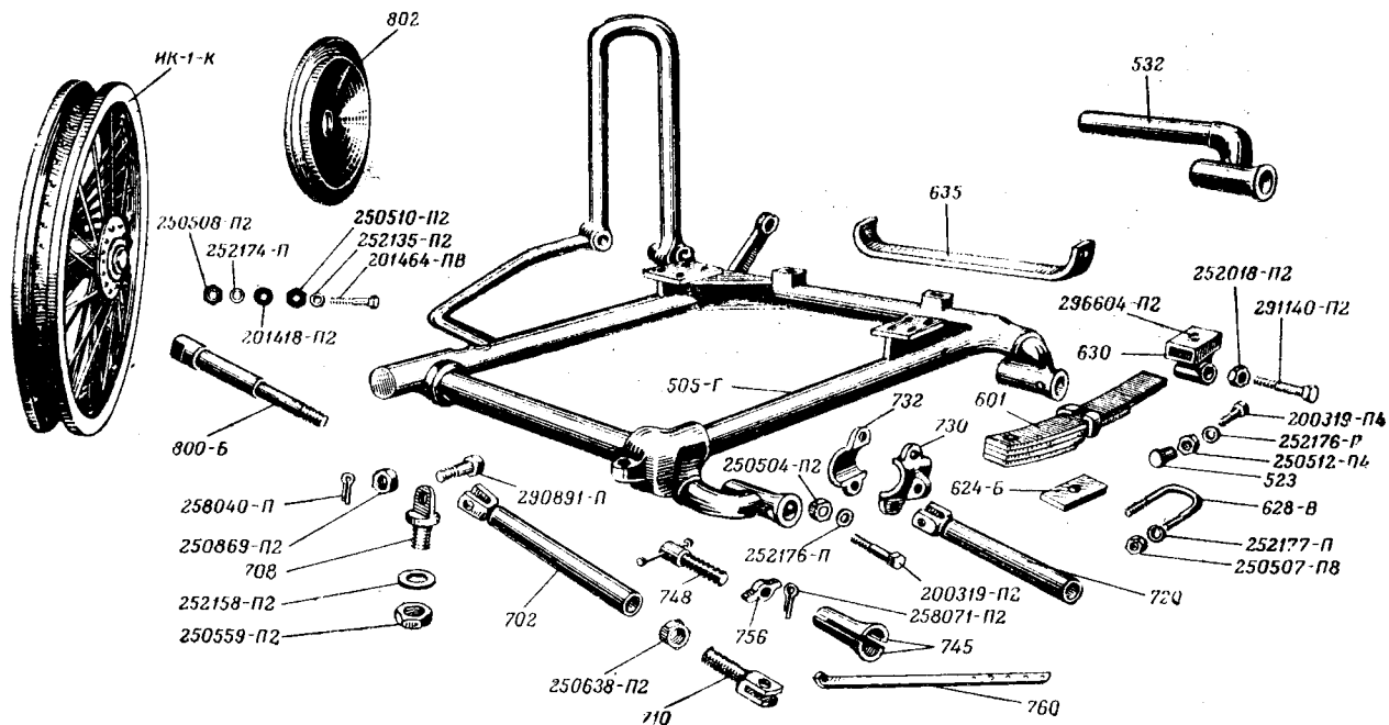
Рис. 18 ШАССИ КОЛЯСКИ
