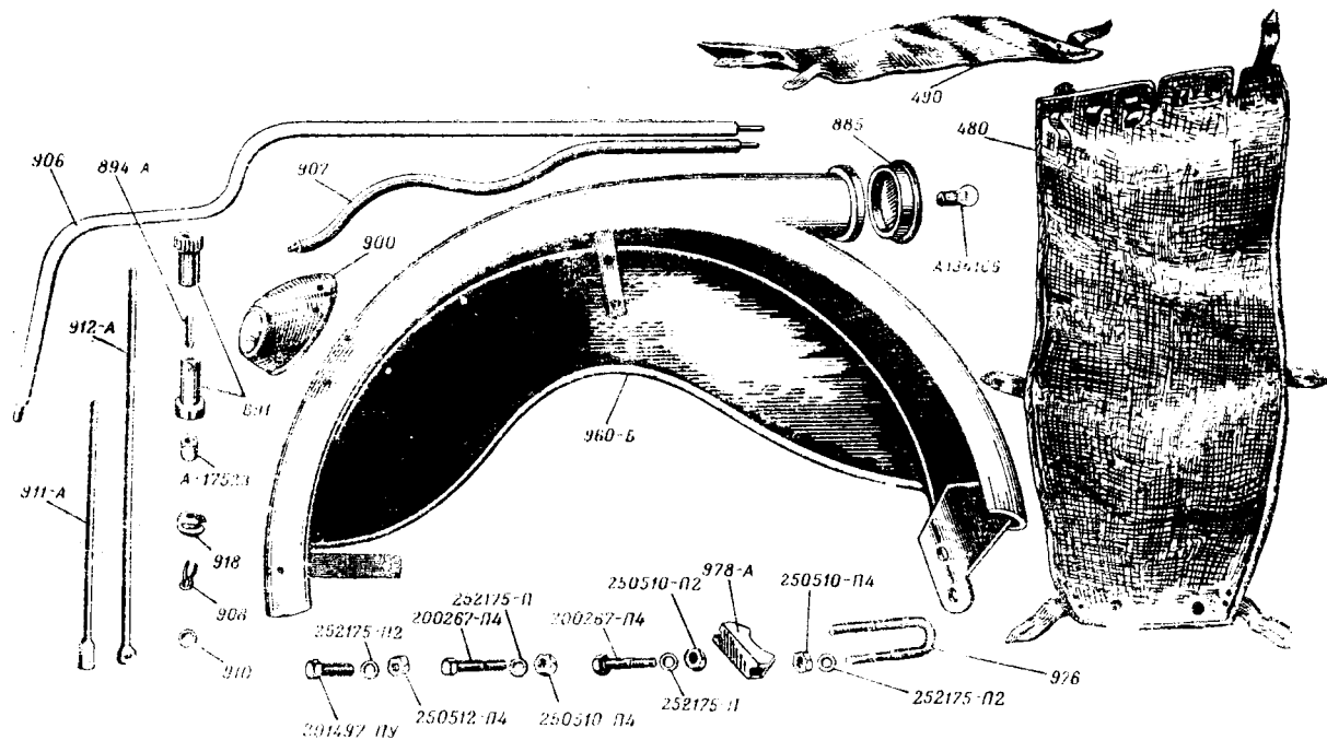
Рис. 17 ШАССИ КОЛЯСКИ
