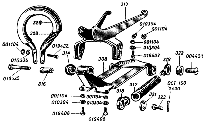
Рис. 12 ГРУППА 7214. СЕДЛО ЗАДНЕЕ
